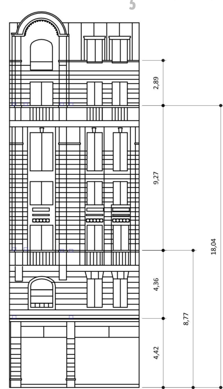
DET1 DETALHAMENTO DA FACHADA EDIFÍCIO ZICO
