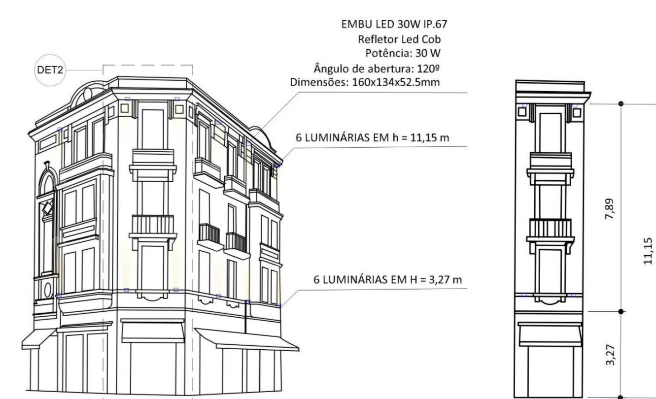
PERSPECTIVA EDIFÍCIO N° 628, AV. SÃO JOÃO ALOCÇÃO DOS PONTOS DE ILUMINAÇÃO SEM ESCALA
